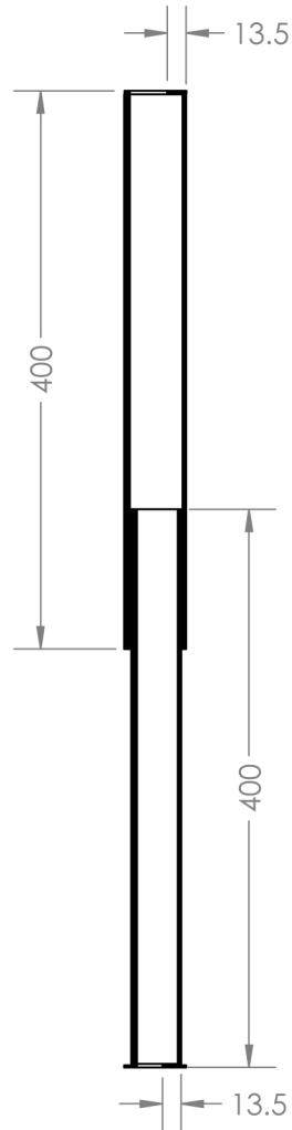
SECTION A-A SCALE 1 : 6
